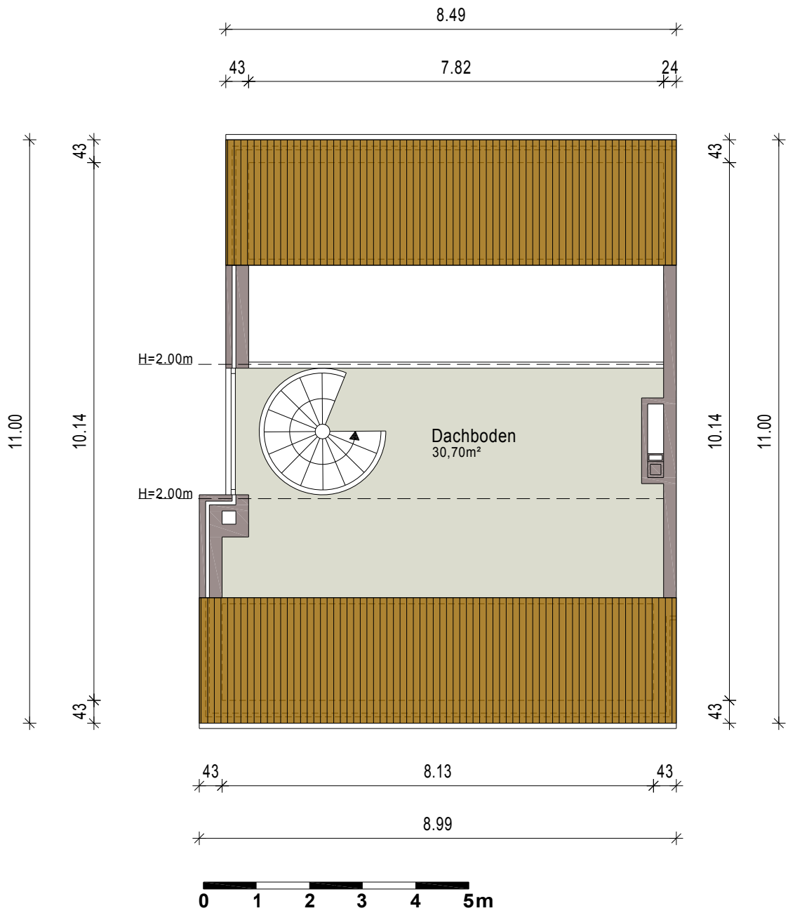
Dachgeschoss
