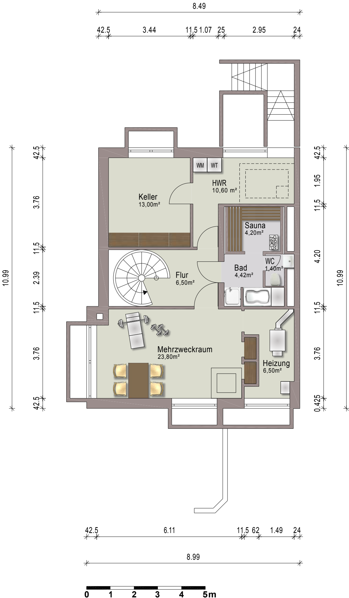
Kellergeschoss
