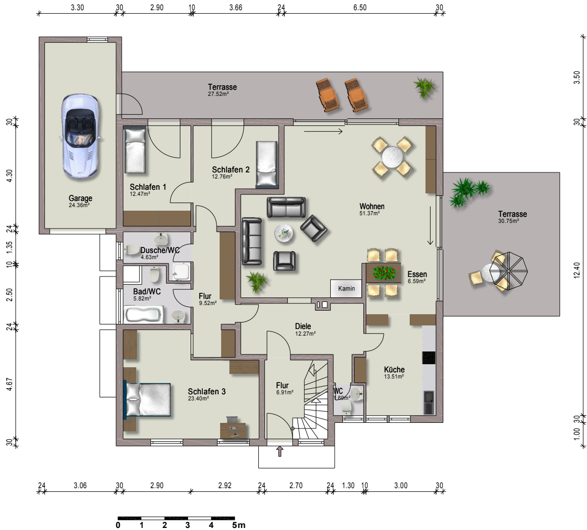
Erdgeschoss
