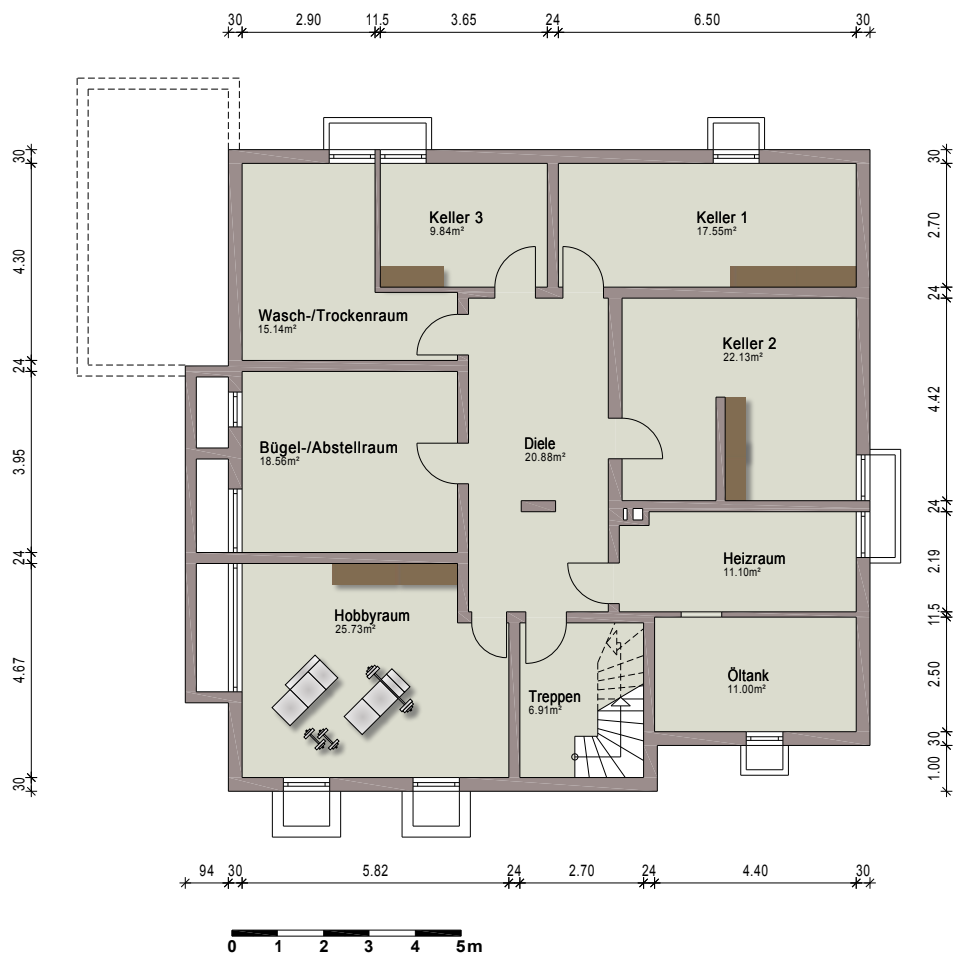
Kellergeschoss
